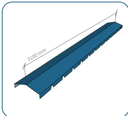
Fecho de canto P5G
