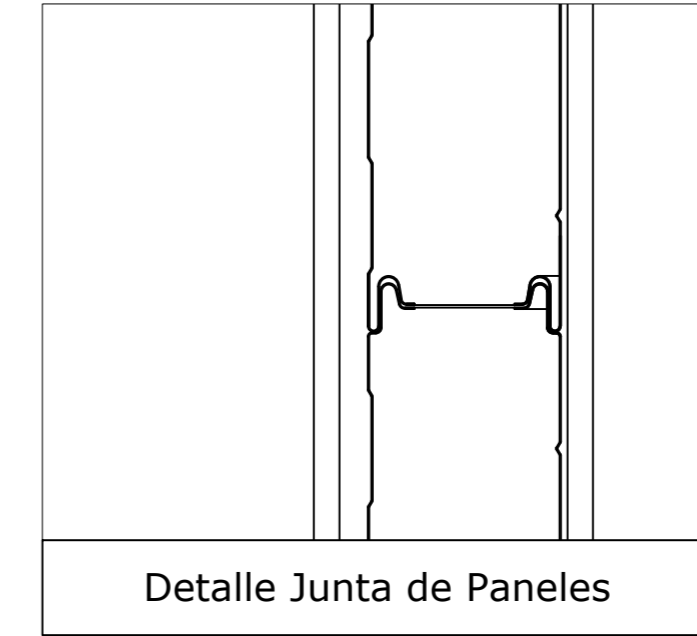
Detalle Junta de Paneles
