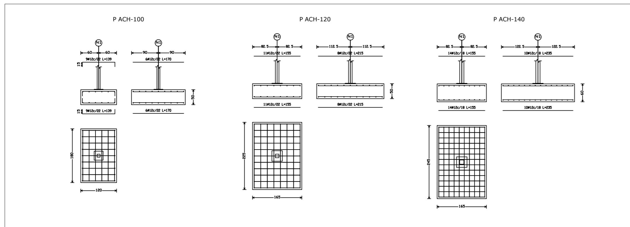
Pantalla Acústica ACH - Cimentaciones
