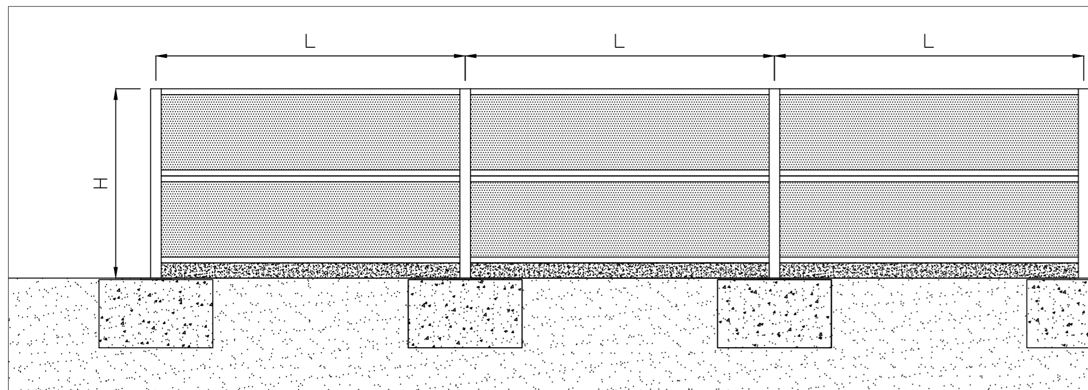
Alzado Pantalla Acústica ACH - Cara fonoabsorbente
