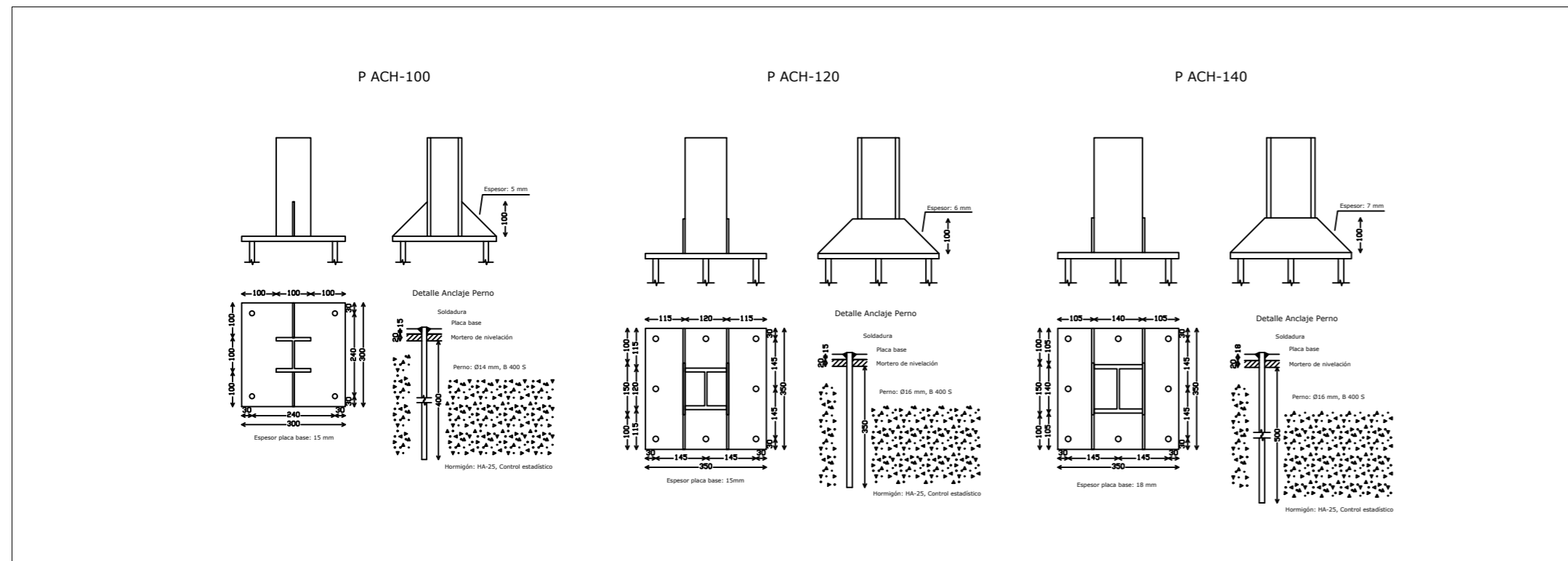
Pantalla Acústica ACH - Placas de anclaje
