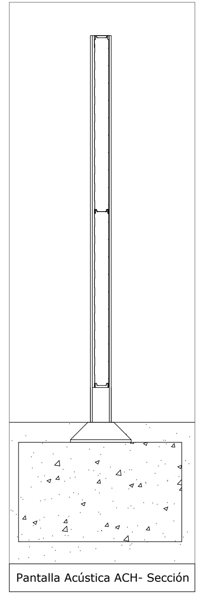
Pantalla Acústica ACH- Sección
